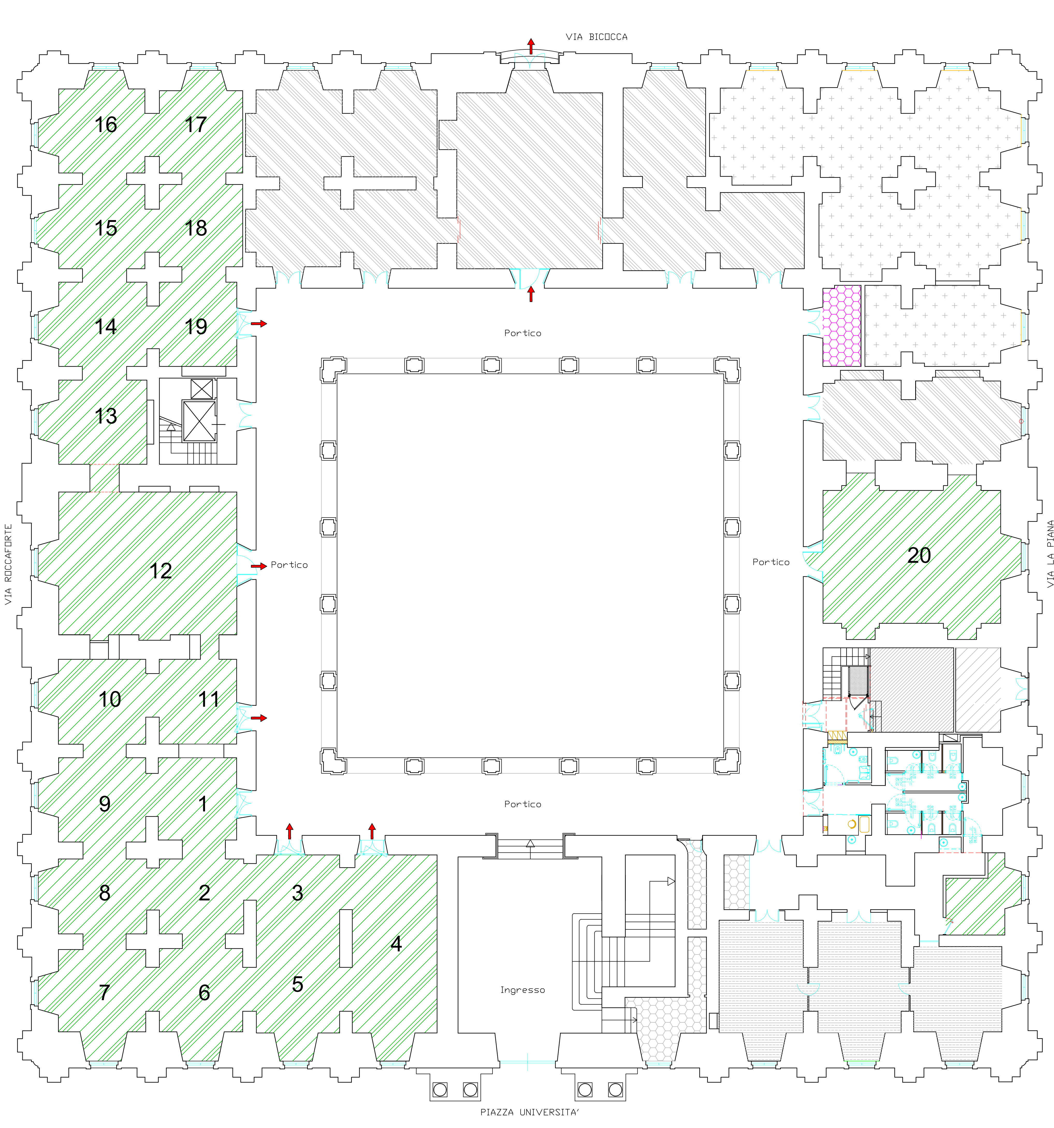
PALAZZO CENTRALE stato di fatto, piano terra scala 1:100
