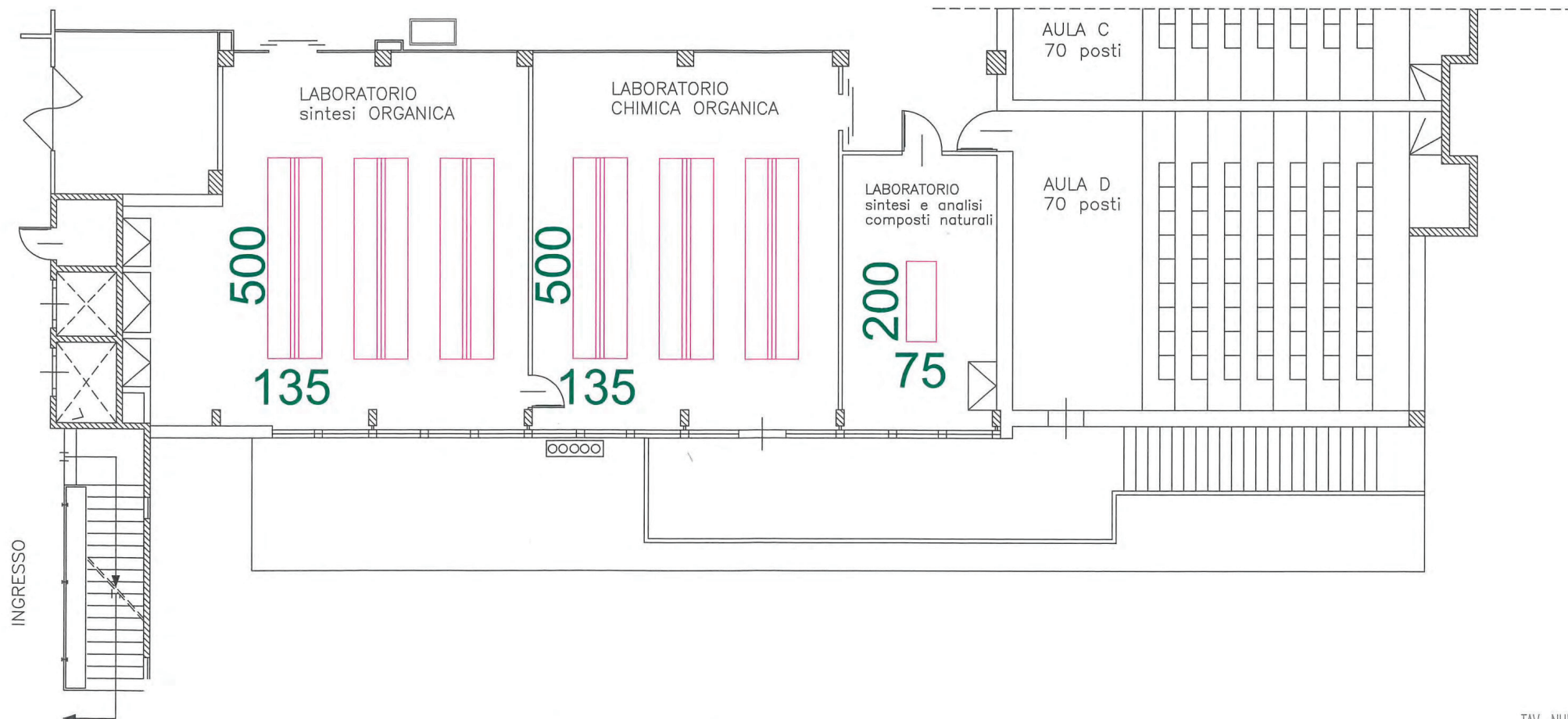
EDIFICIO 1 - CORPO A PIANO TERRA
