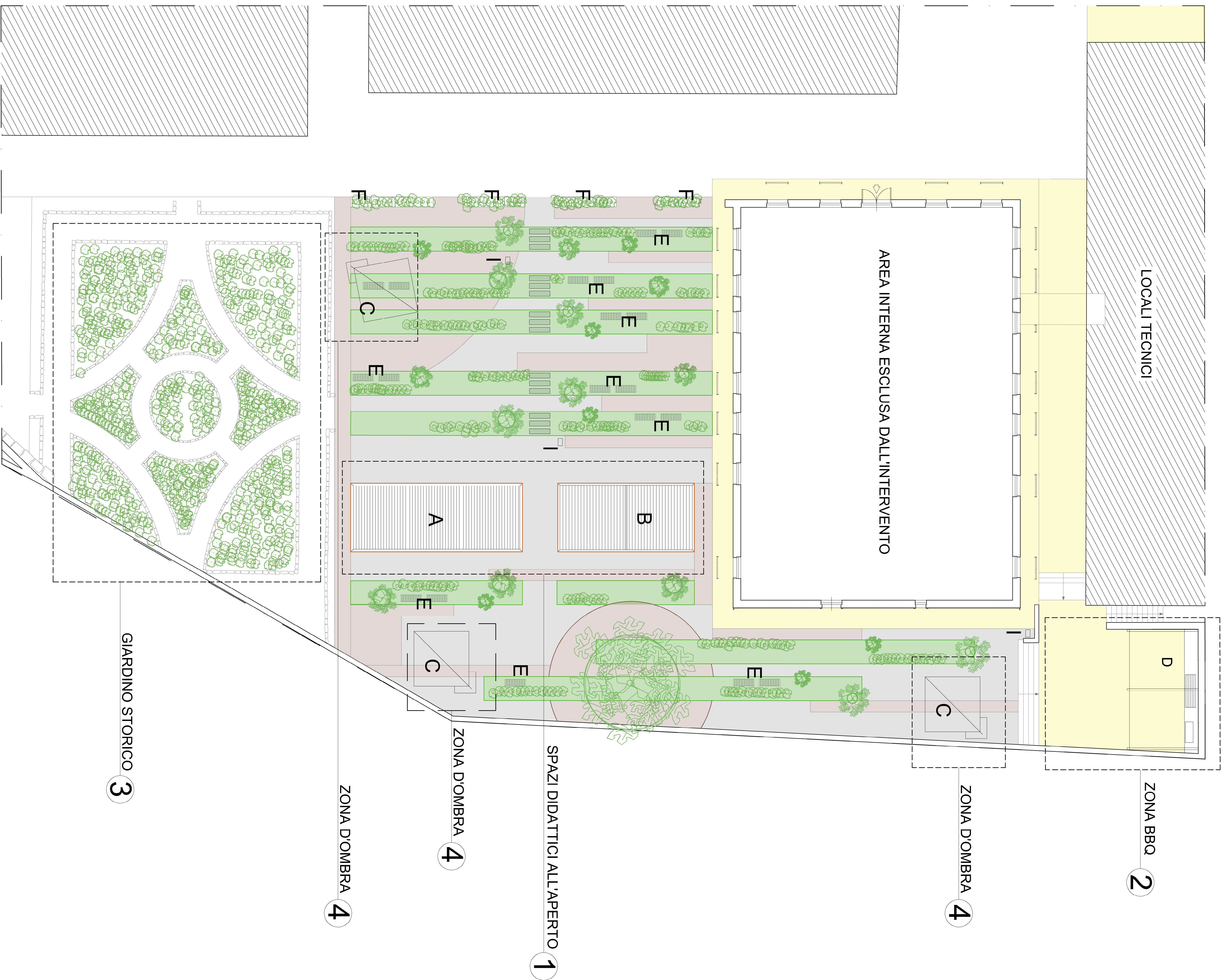
PLANIMETRIA INTERVENTO - SCALA 1:100
