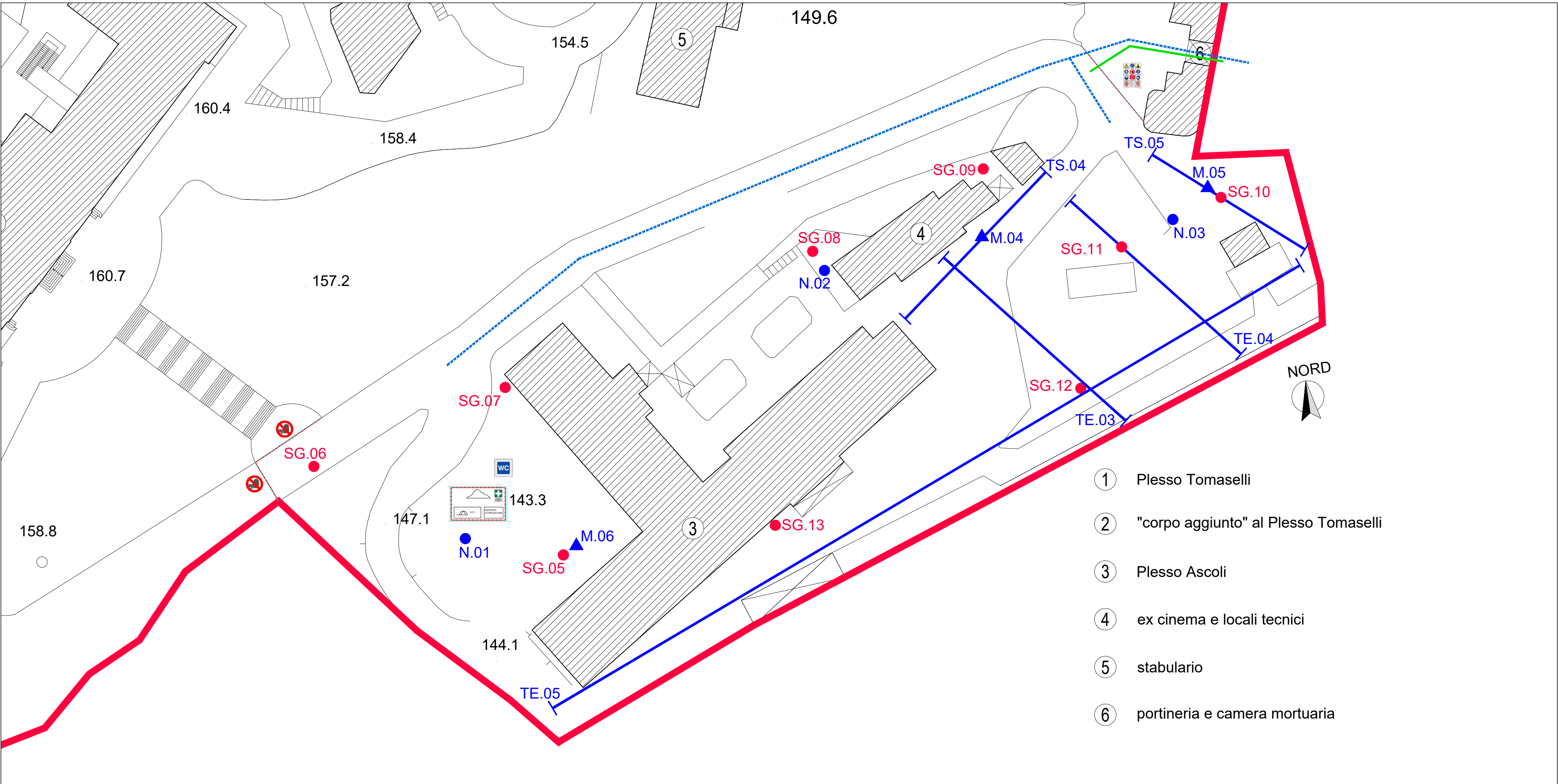
PLANIMETRIA GENERALE STATO DI FATTO - PLESSO ASCOLI scala 1:500
