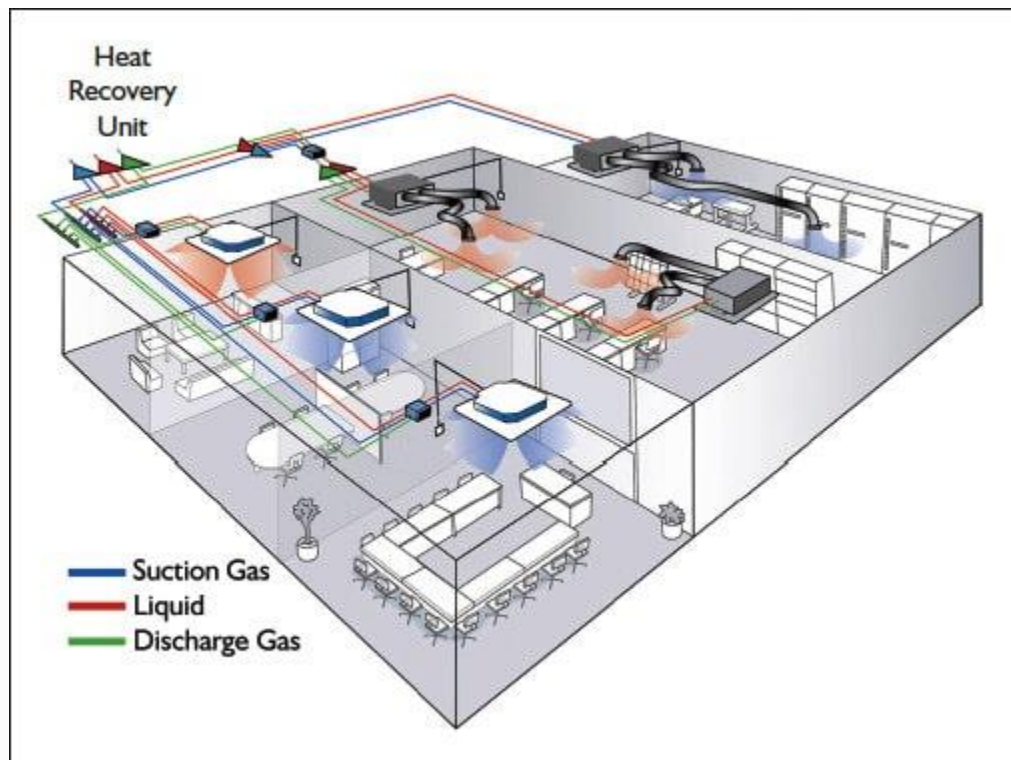
• Sistema “Tipo” di un impianto VRF (solo indicativo)
